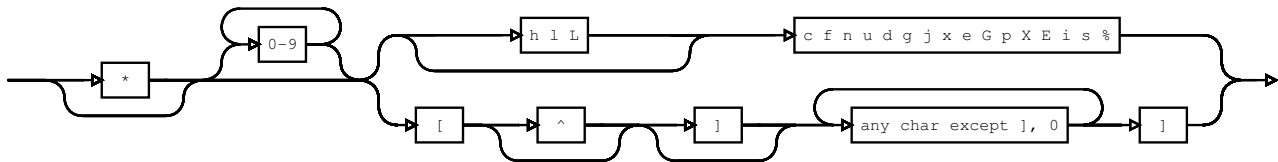
Рис. 2: Синтаксис спецификаций преобразования функции scanf (C90)
